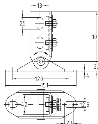
Инсталиране на конзоли в сводове или в кръгли канали и шахти за кабели
