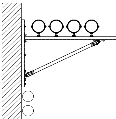
Тръби, монтирани върху MPC конзола с диагонална подпора
