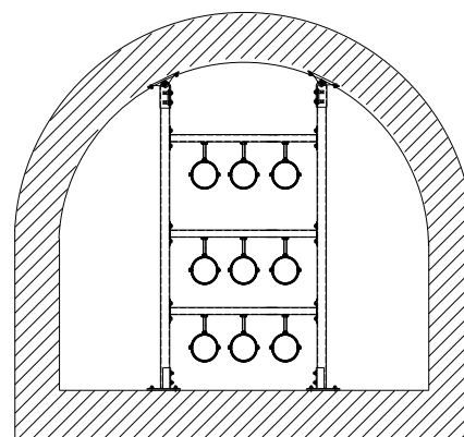
Инсталиране на конзоли в сводове или в кръгли канали и шахти за кабели
